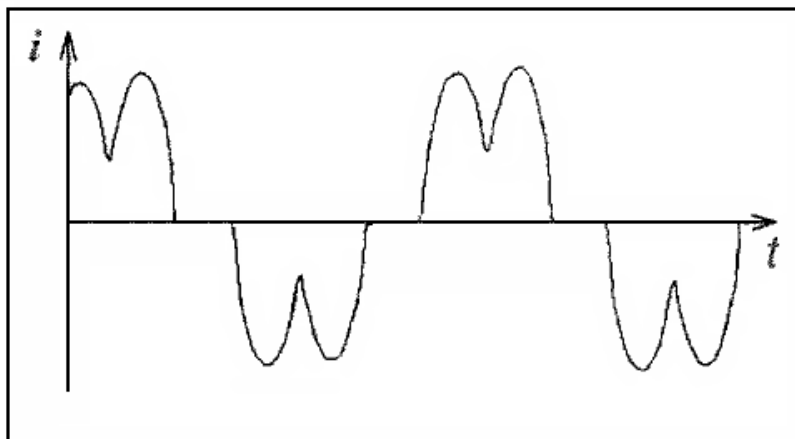
Рис.2. Форма тока трехфазного выпрямителя.
