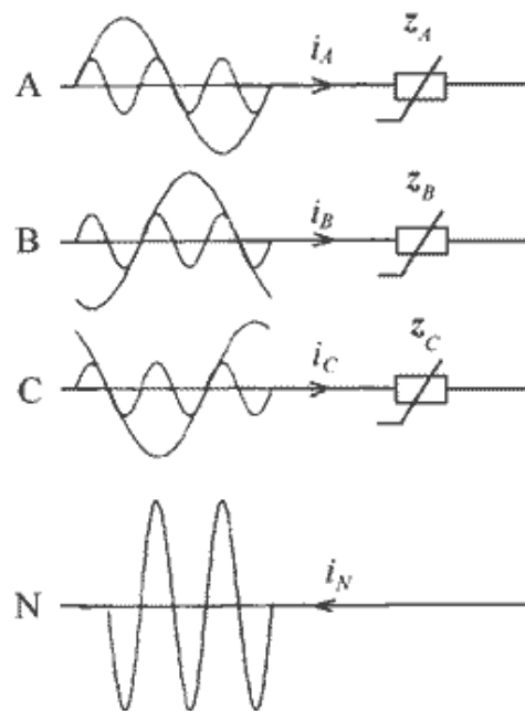
Рис.5. Процесс формирования тока нейтрали при нелинейной нагрузке.
